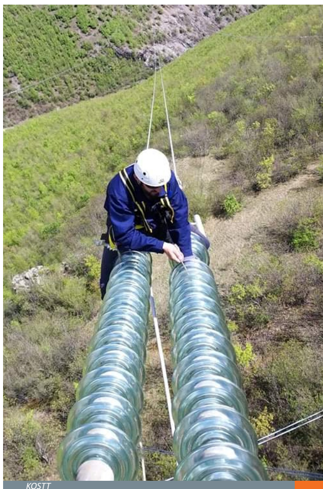
Pamje nga punimet në linjën interkonektive 400 kV LP 4372 që lidhë Nënstacionin 400/110 kV Peja 3 me NS Ribarevina (Mali i Zi) 1
